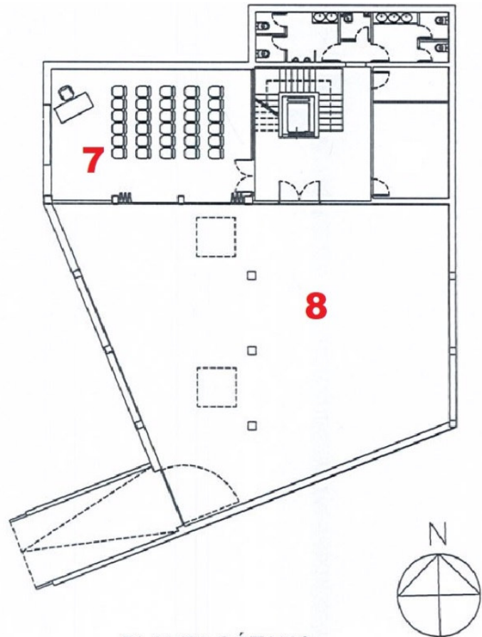
PLANTA SÓTANO
